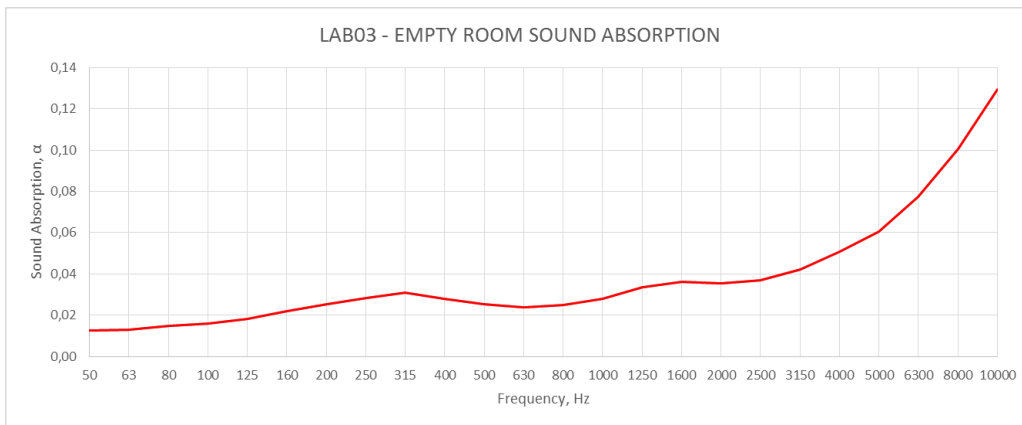
Şekil 5. LAB-03 Boş durumda çınlama süresi ölçümleri ve toplam oda içi yutuculuk düzeyi hesaplama sonuçları
