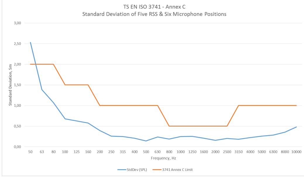
Şekil 8. LAB-03 içerisinde Referans ses kaynağı (RSS) ile TS EN ISO 3741 EK.C'ye göre yapılan ölçüm sonucunda standart sapma limit değerlerine göre değerlendirmesi
