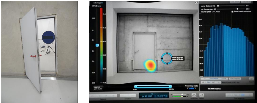
Şekil 3. Akustik kamera kullanımı ile kapı sisteminin ses yalıtım zayıflıkları veya kaçak olan bölgelerin belirlenmesi
