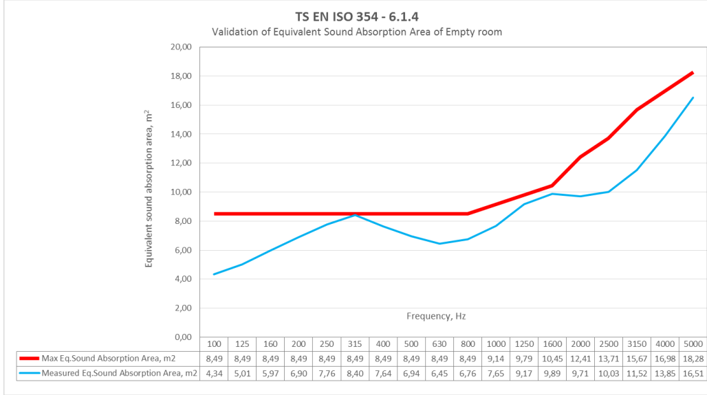
Şekil 6. LAB-03 Boş durumdaki yutuculuk değerlerinin TS EN ISO 354 Madde 6.1.4 ile doğrulama sonuçları
