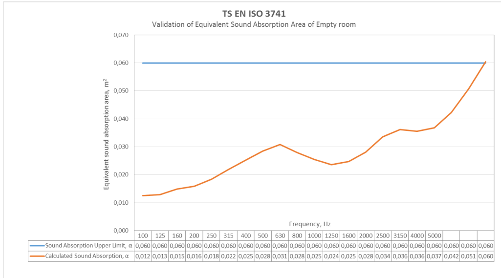
Şekil 7. LAB-03 ses gücü düzeyi ölçümleri için yerleştirilen ses yutucu panellerden sonra TS EN ISO 3741 uyarınca toplam yutucu yüzey doğrulaması
